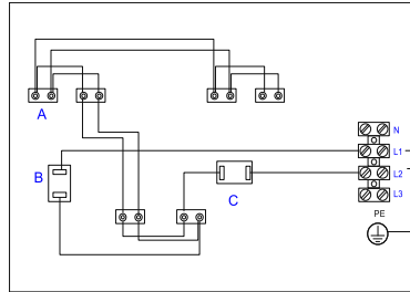
2~ 400V jungimo schema 2~ 400V electrical connection 2~ 400В электрическое подключение 2 ~ 400V elektrischer Anschluss
