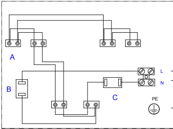
1~ 230V jungimo schema 1~ 230V electrical connection 1~ 230В электрическое подключение 1 ~ 230V elektrischer Anschluss
