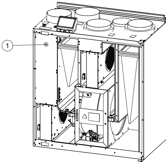
Pav. 6 Apsaugos nuo perkaitimo paleidimo iš naujo mygtukas
